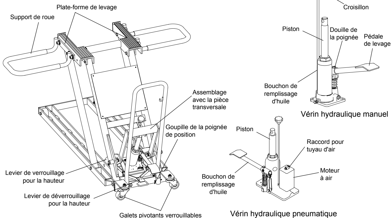
Figure 1 : Pièces des lève-tondeuses T-5750
