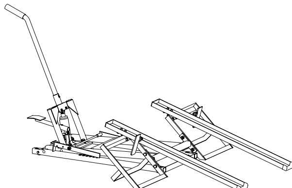
Figura 6: Ensamblaje final
