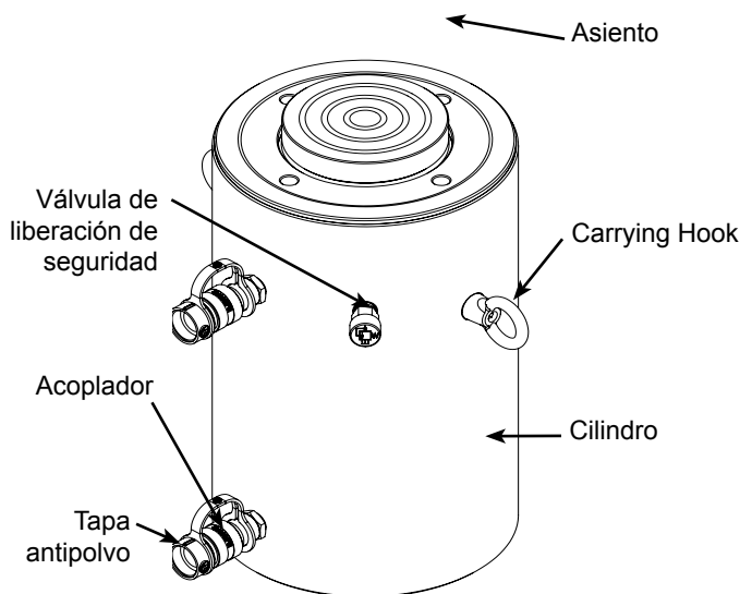
Figura 1: Componentes habituales del cilindro
