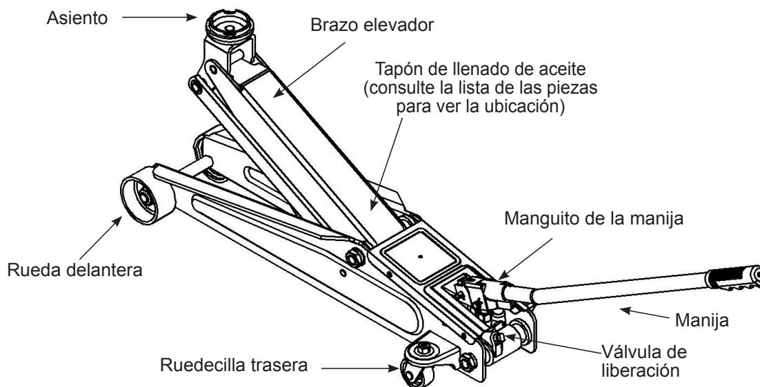
Figure 1 - Nomenclatura habitual de un gato de piso
