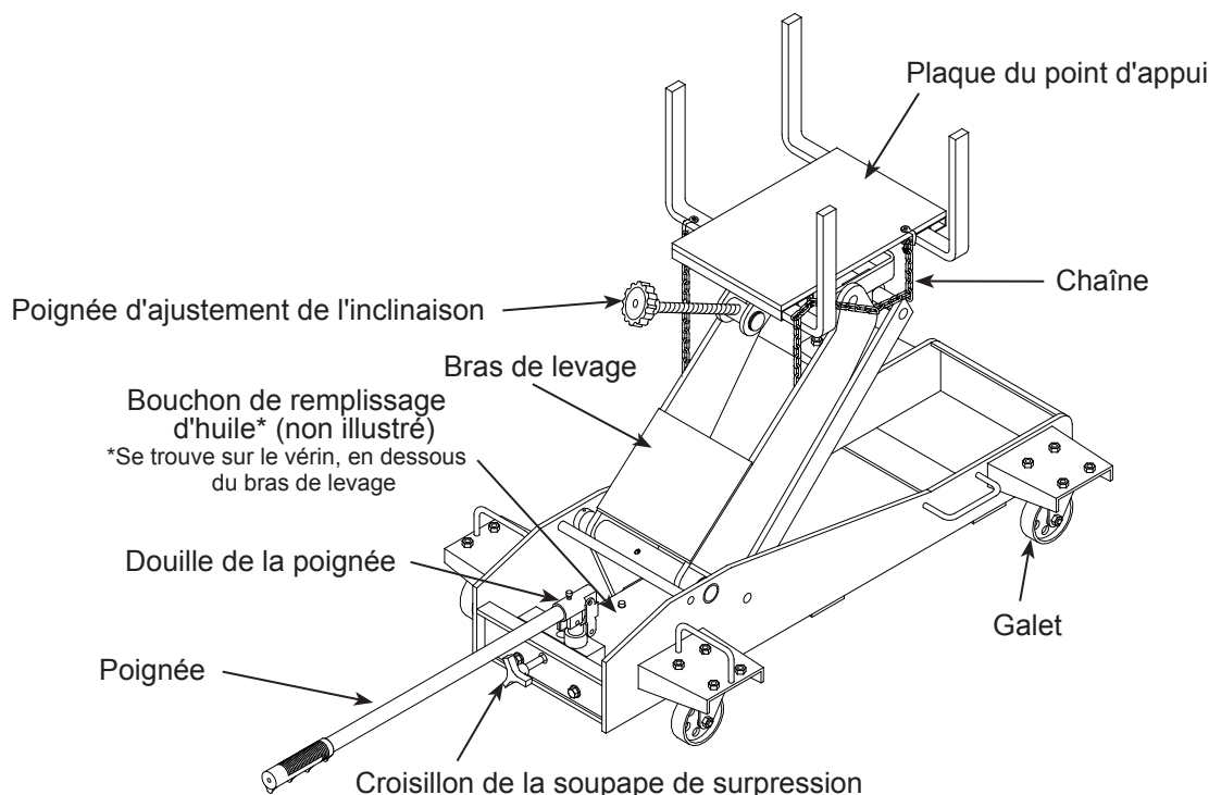
Figure 1 - Composants types d'un cric pour transmission
