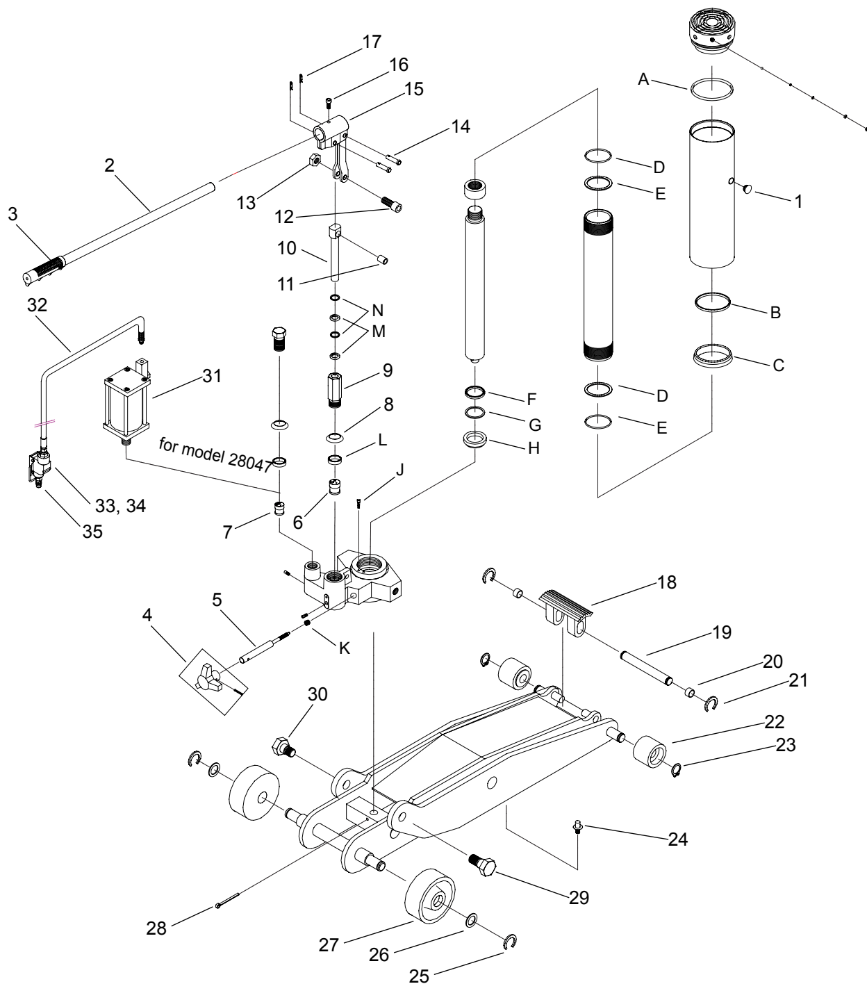
Figure 2 : Illustration des pièces de rechange des modèles 28045 et 28047
