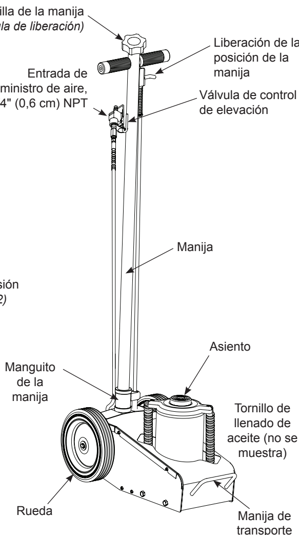
Figura 1: Nomenclatura del modelo 23301
