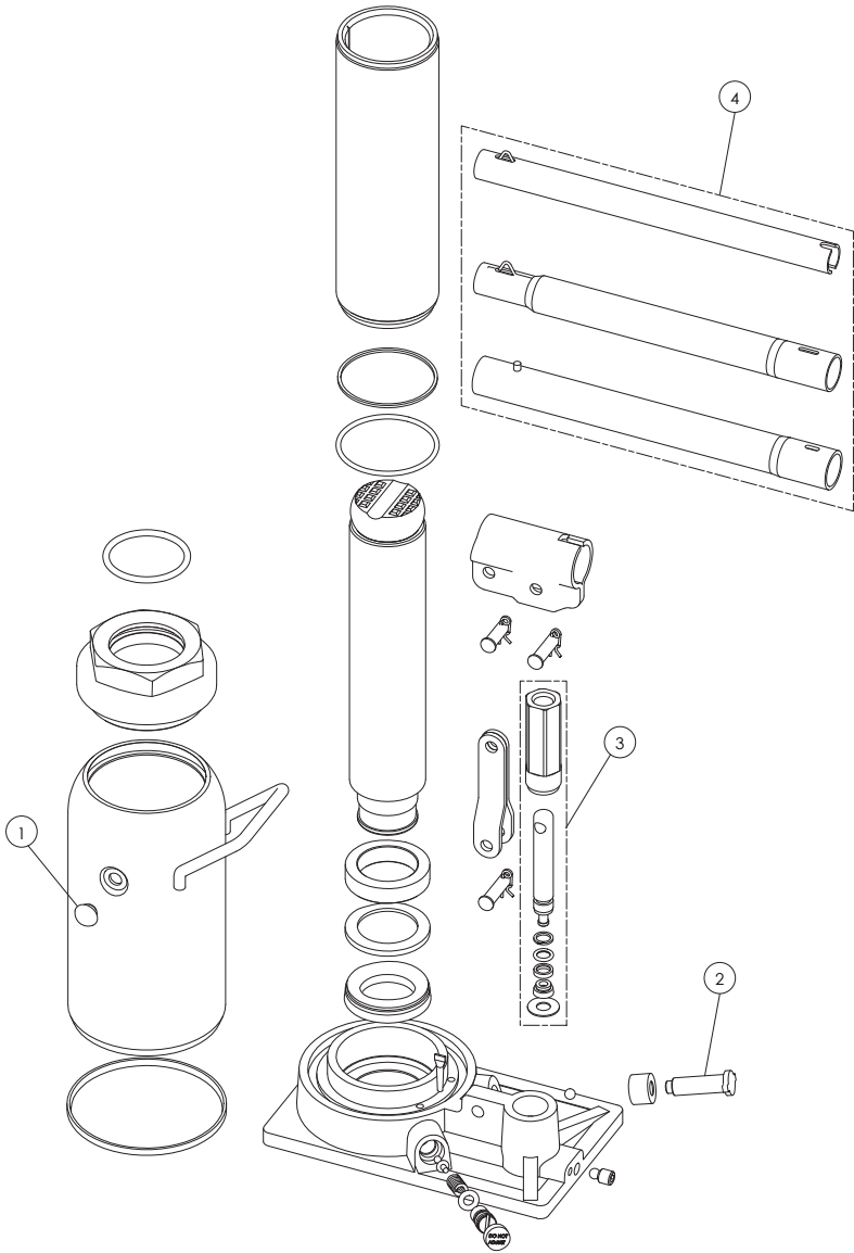
Figura 2: Ilustración de piezas de repuesto para los modelos 10120, 10128, 10200 y 10208 Piezas de repuesto para los modelos 10120, 10128, 10200 y 10208
